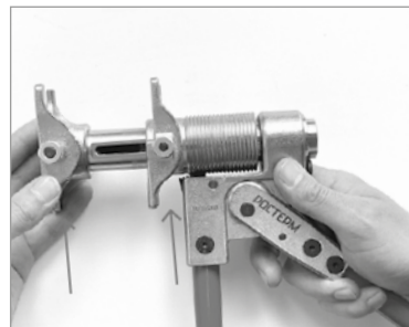
5. Переведите ручку тисков в верхнее положение, потяните вниз блокиратор, чтобы разъединить рычаг и насадку на тиски, вытаскивайте осевые болты, установите необходимую насадку на тиски, зафиксируйте осевой болт и верните в исходное положение блокиратор
